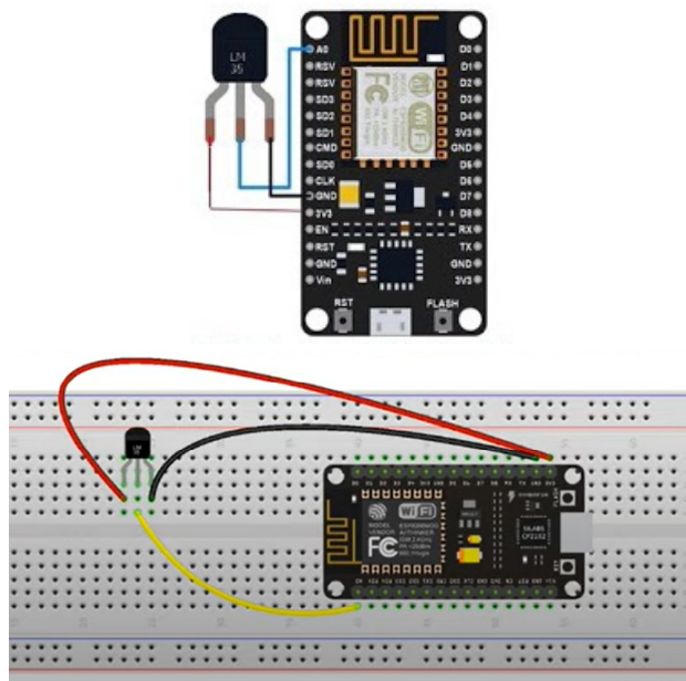
Figura 2. Esquema de cómo interconectar el LM35 al NodeMCU ESP8266
