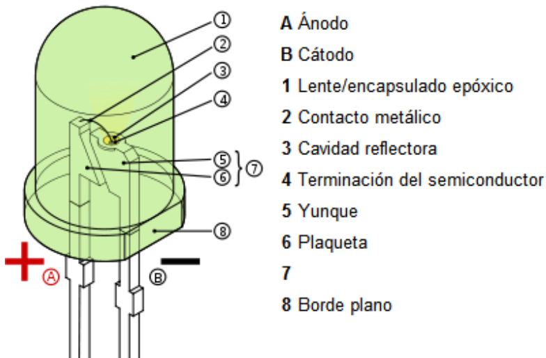
Figura 4. Partes de un LED
