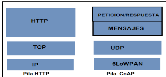
Figura 8. Pila de protocolo HTTP y pila de protocolo CoAp
