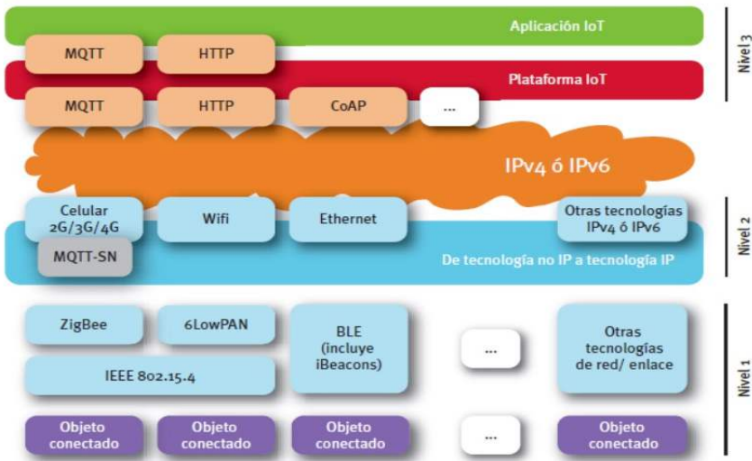
Figura 2. Arquitectura de tres niveles - objetos conectados sin protocolo IP
