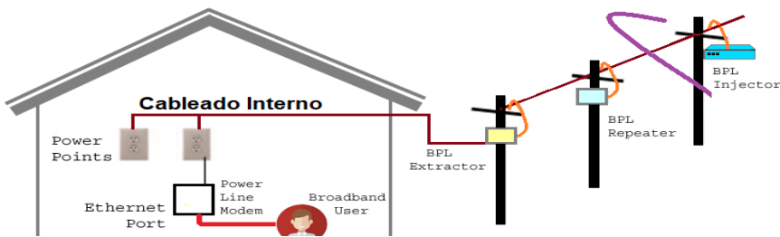
Figura 4. Sistemas PCL
