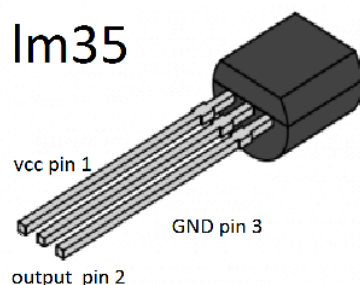
Figura 2. Sensor de temperatura LM35
