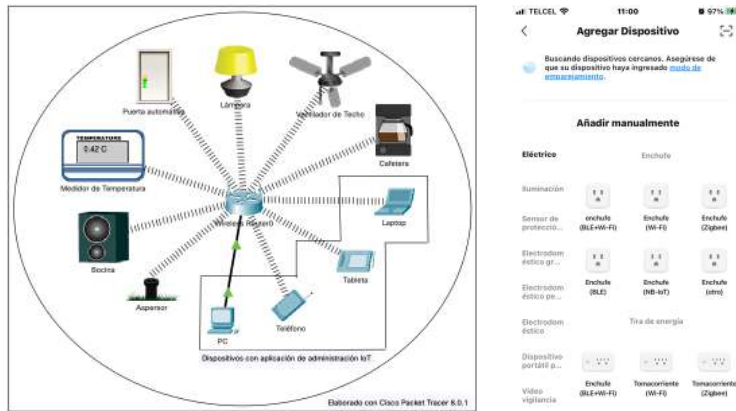
Figura 1. Escenario IoT con dispositivos integrados y aplicación de administración
