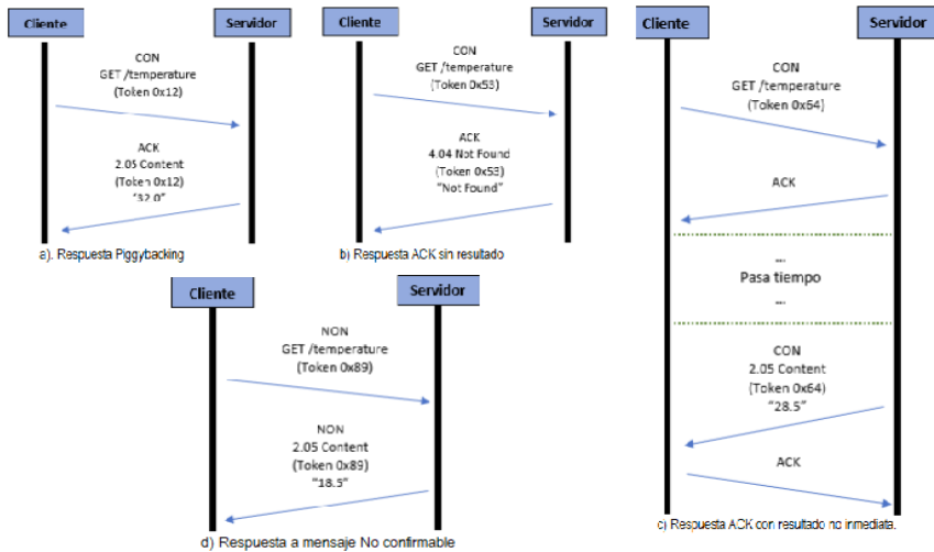
Figura 9. Tipos de respuestas a mensajes confirmables y no confirmables CoAp
