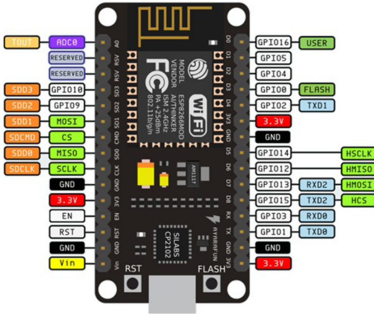
Figura 6. Distribución de los pines GPIO del NodeMCU ES8266
