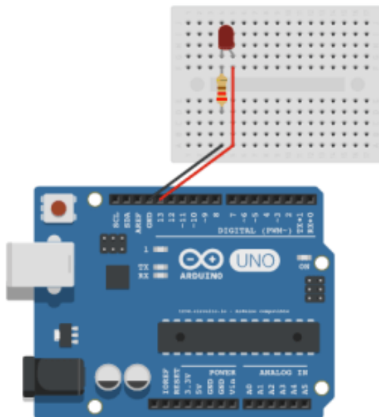
Figura 5. Esquema de cómo debe montarse el circuito para poder prender y apagar el LED con la placa Arduino
