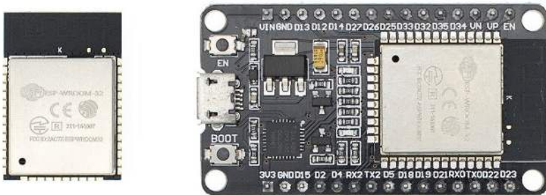
Figura 3. Diferencias físicas entre un módulo de microcontrolador y una placa de desarrollo
