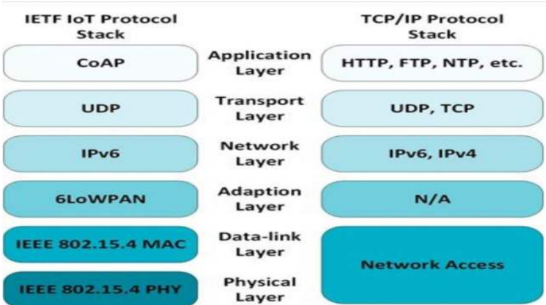
Figura 6. Comparativa de la Suite TCP/IP y la pila de protocolos IoT
