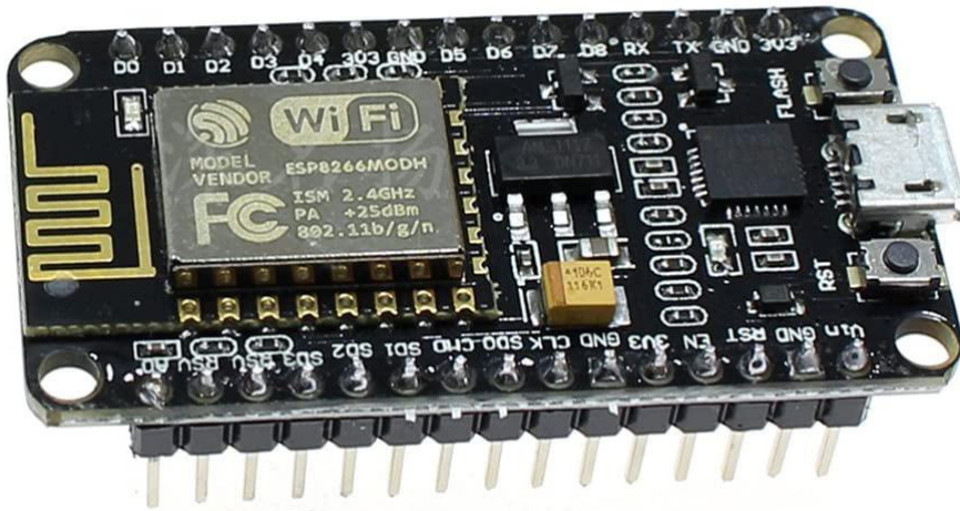
Figura 2. Placa de desarrollo IoT que utiliza el microcontrolador ESP8266
