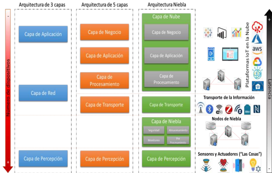
Figura 1. Arquitecturas IoT Relevantes
