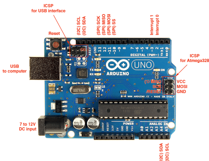
Figura 1. Placa Arduino UNO
