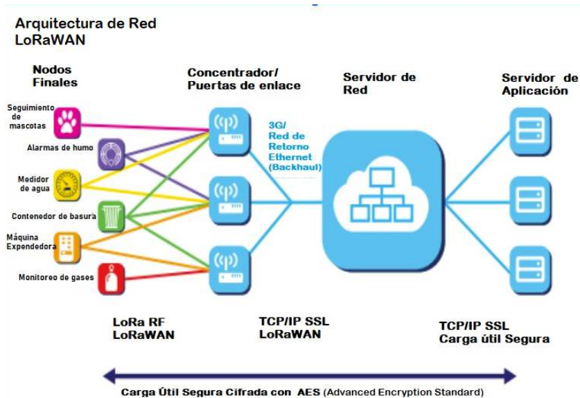
Figura 5. Arquitectura de una red LoRaWAN
