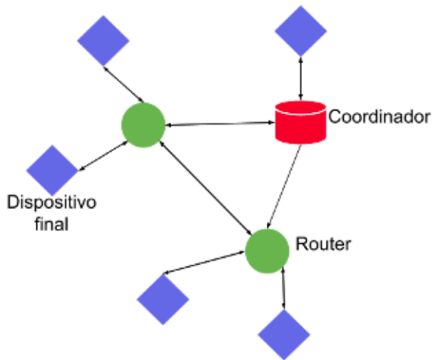
Figura 4. Red de malla Zigbee
