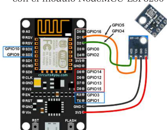
Figura 1. Sensor BMP180 y su interconexión con el módulo NodeMCU ESP8266
